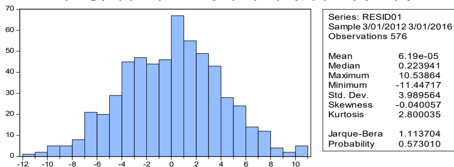
نمودار ۱. نمودار هیستوگرام و آماره جارگ برای باقیمانده در مدل رگرسیونی شماره (۱)
