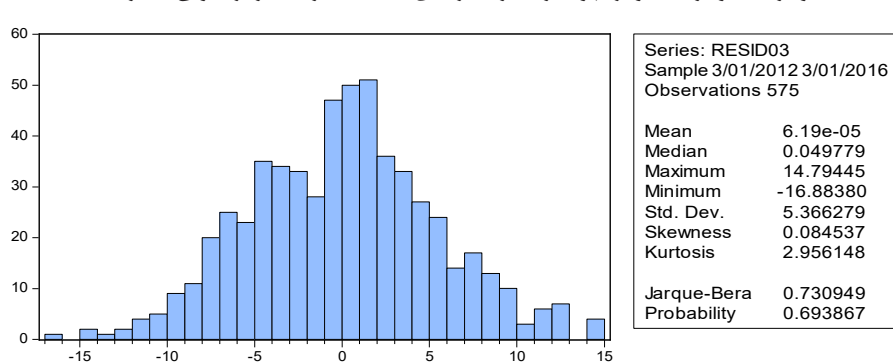
نمودار ۳. نمودار هیستوگرام و آماره جارگ برای باقیمانده در مدل رگرسیونی شماره (۳)
