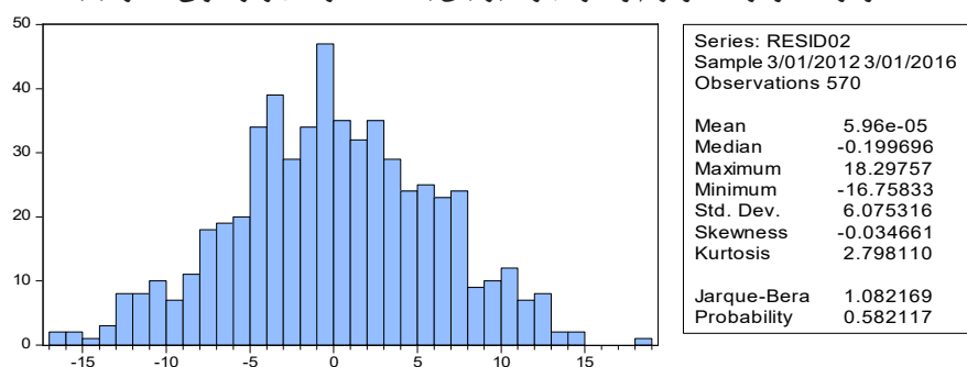
نمودار ۲. نمودار هیستوگرام و آماره جارگ برای باقیمانده در مدل رگرسیونی شماره (۲)
